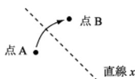
図3 上: xl = m 中: l = xm 下: xA = B
