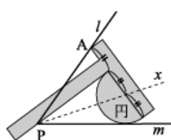
図1 超定規。任意角Pの l が A を通り、 m が円に接するように定規を当てると x が角を三等分する。
