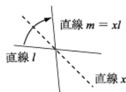
図2 折紙作図の公理系 折り線の本質は対称移動。矢印は逆向きも考える。図示した破線以外の直線 x が存在
